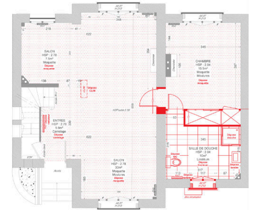
Plan de démolition RDC
