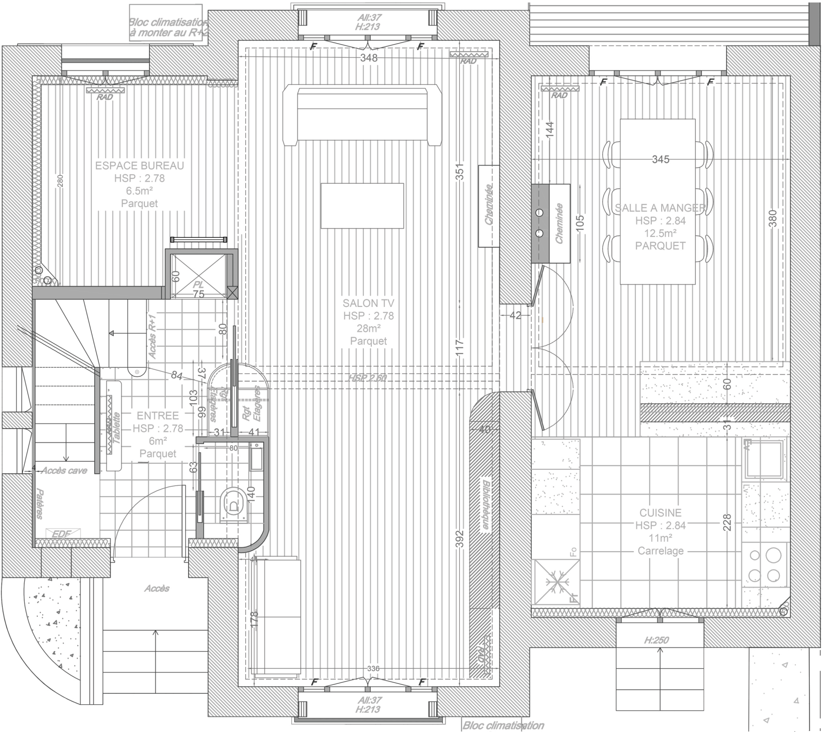
Plan projet RDC (isolation) - Mise en valeur des lignes courbes Échelle 1/50e
