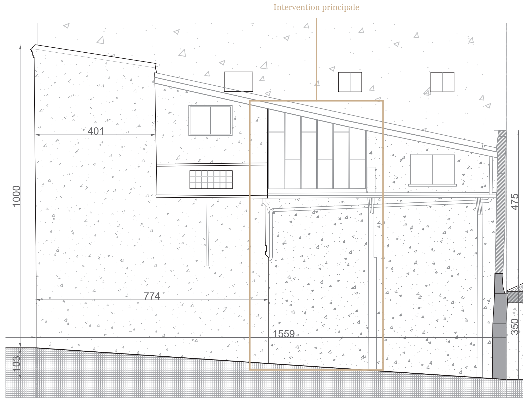
Coupe de l'existant avant intervention - Ouverture en verrière Échelle 1/50e
