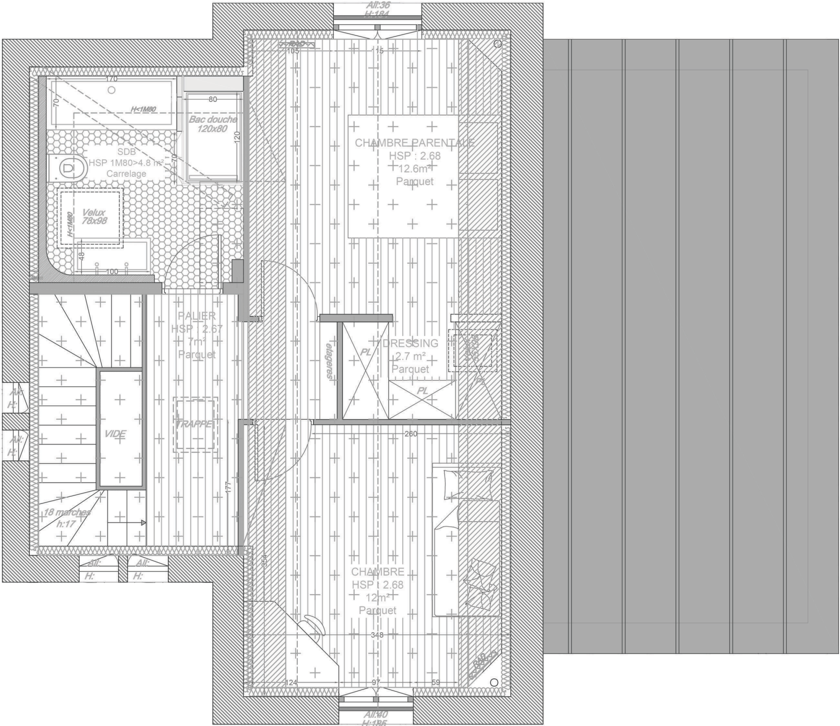
Plan projet R+2 (isolation) - Ouverture des espaces Échelle 1/50e
