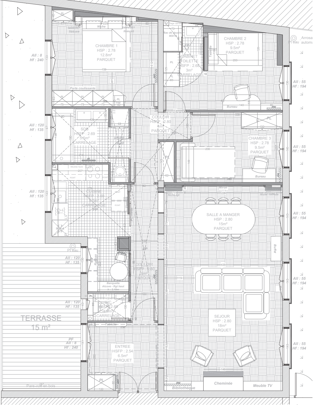
Plan de projet - Réorganisation des espaces Échelle 1/50e
