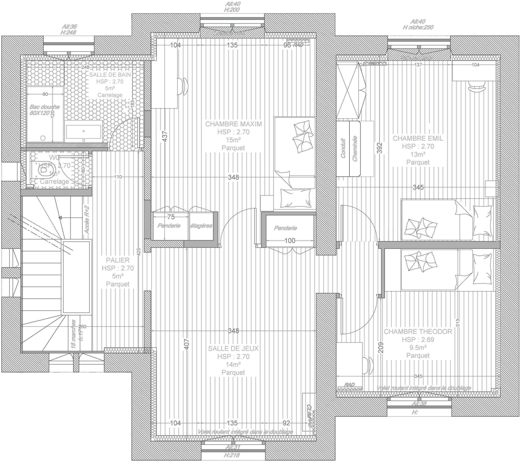
Plan projet R+1 (isolation) - Séparation des espaces de nuit Échelle 1/50e
