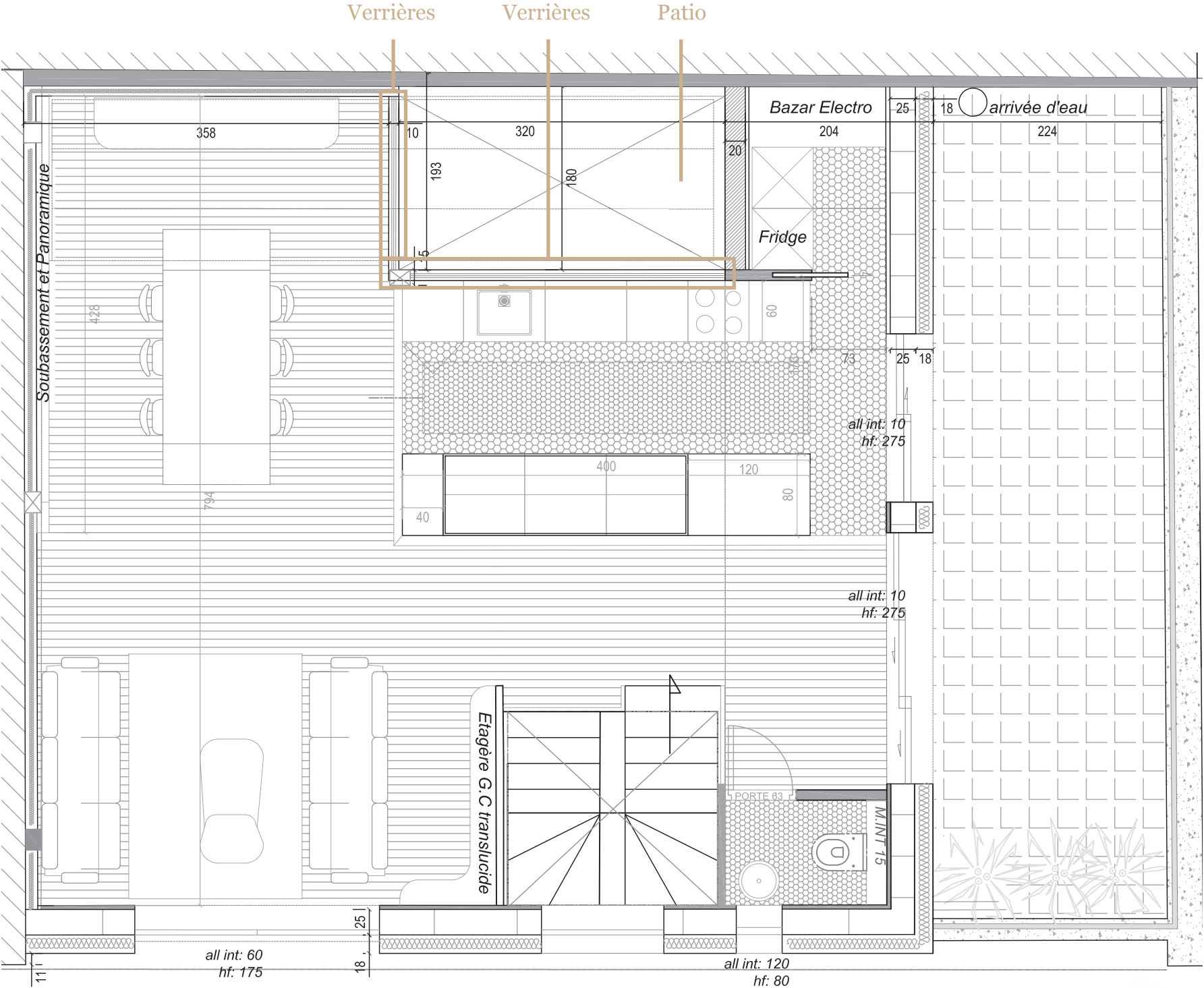
Plan projet R+2 — Espaces de vie ouverts Échelle 1/50e
